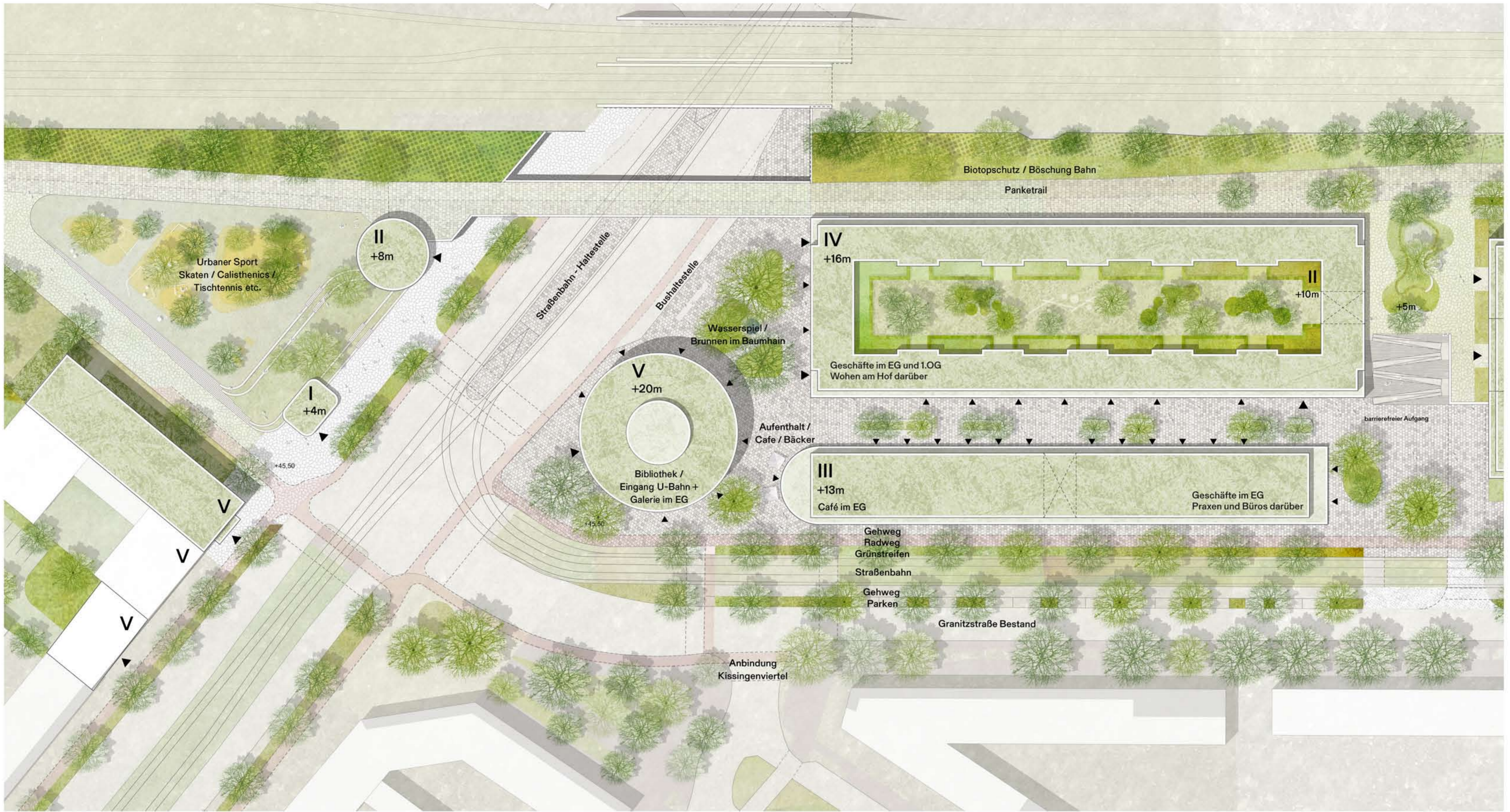
Platz an der Berliner Straße 1:500
